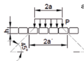
Pflasterdecke (Lastausstrahlung)
