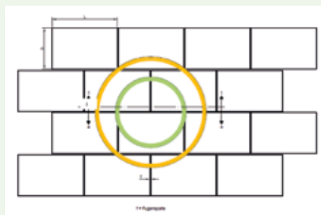
Pflasterdecke (Lastausstrahlung)
